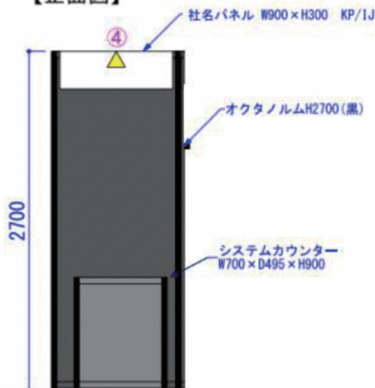
【正面図】
